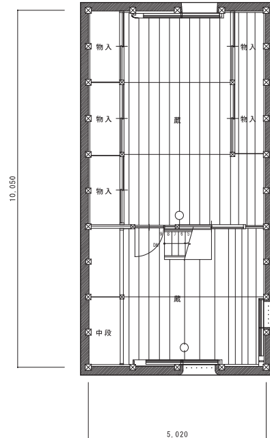
2階平面図
