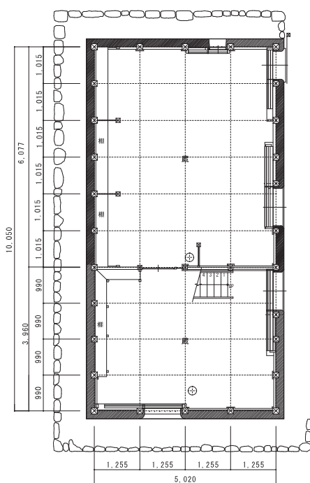
1階平面図
